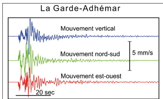
Fig. 4 – En fonction du temps la vitesse du sol enregistrée à la Garde-Adhémar à environ 20 km.
