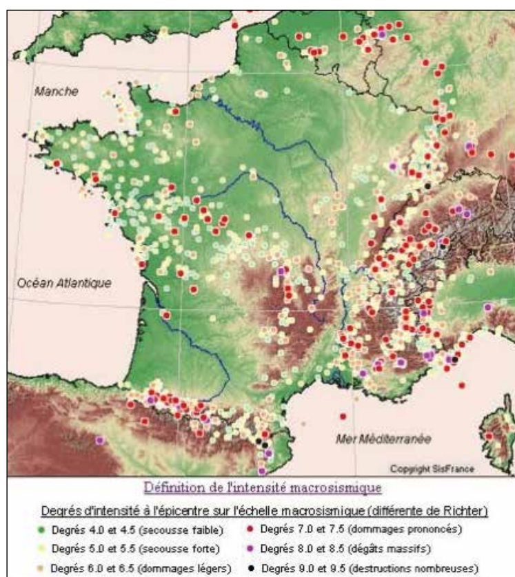
Fig. 1 – Sismicité en France ( SisFrance ) Carte des événements répertoriés sur SisFrance : les points représentent le lieu où est évaluée l'intensité macrosismique la plus importante. Sur la prochaine carte, l'événement du Teil apparaîtra sous la forme d'un point rouge.
