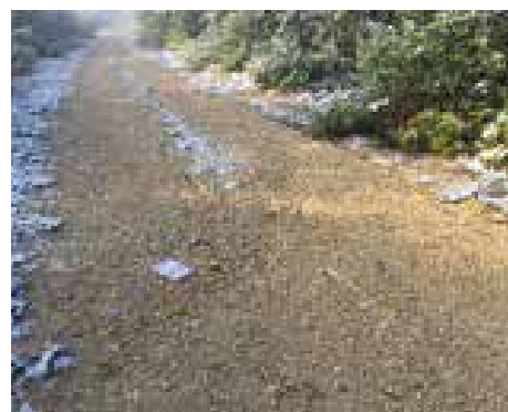
Fig. 3 – photo de traces de surface.
