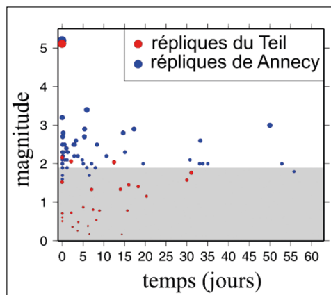
Fig. 5 – Comparaison de l'activité post-sismique entre Annecy (1996) et Le Teil
