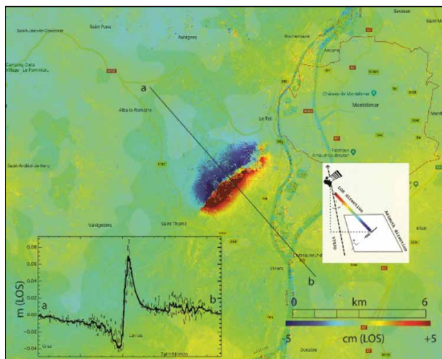
Fig. 2 – Analyse de la déformation du sol par interférométrie radar (InSAR)
